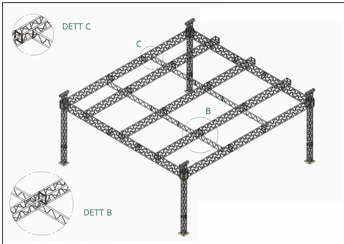
Imagem 2: desenho da estrutura truss
