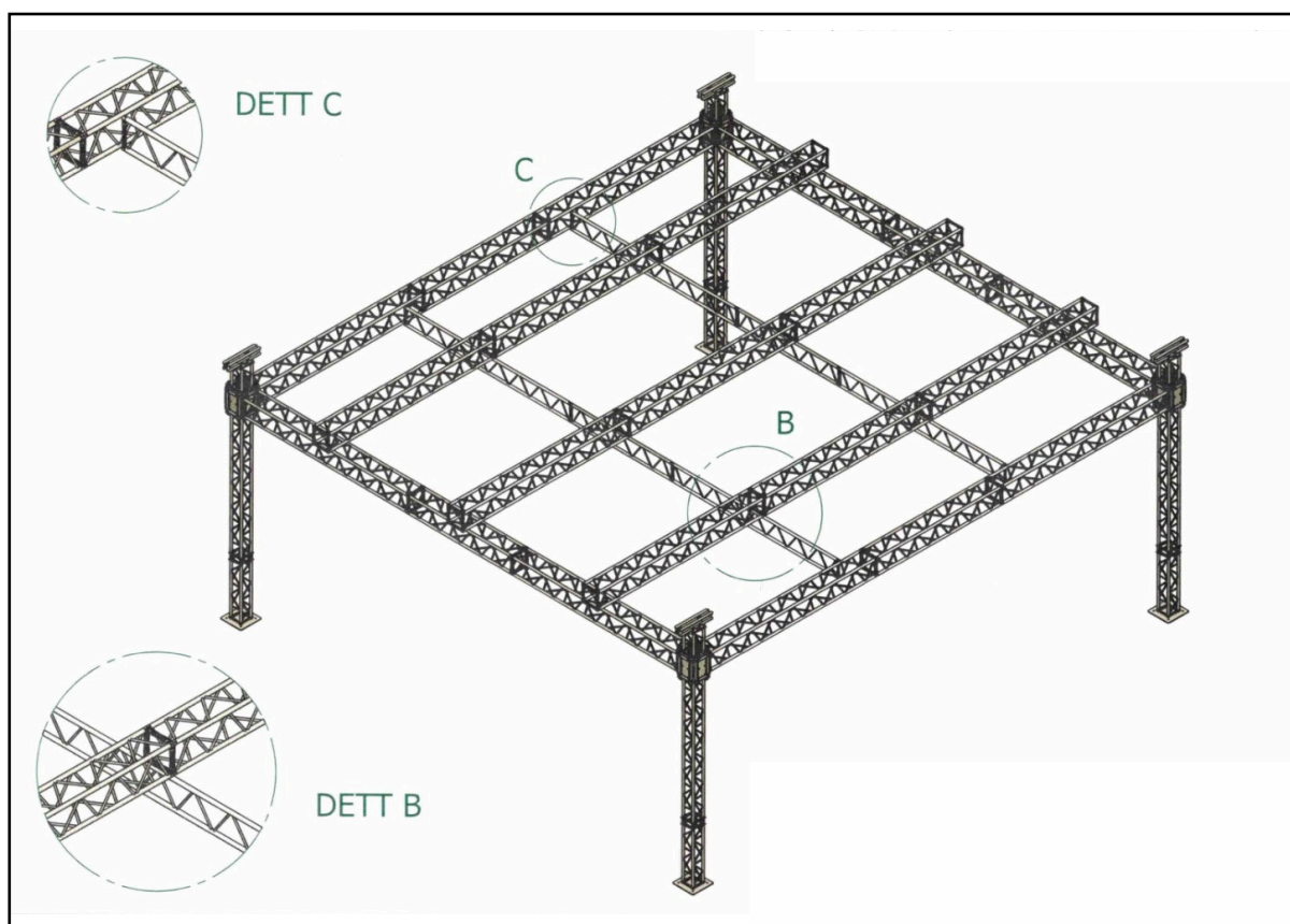
Imagem 2: desenho da estrutura truss
